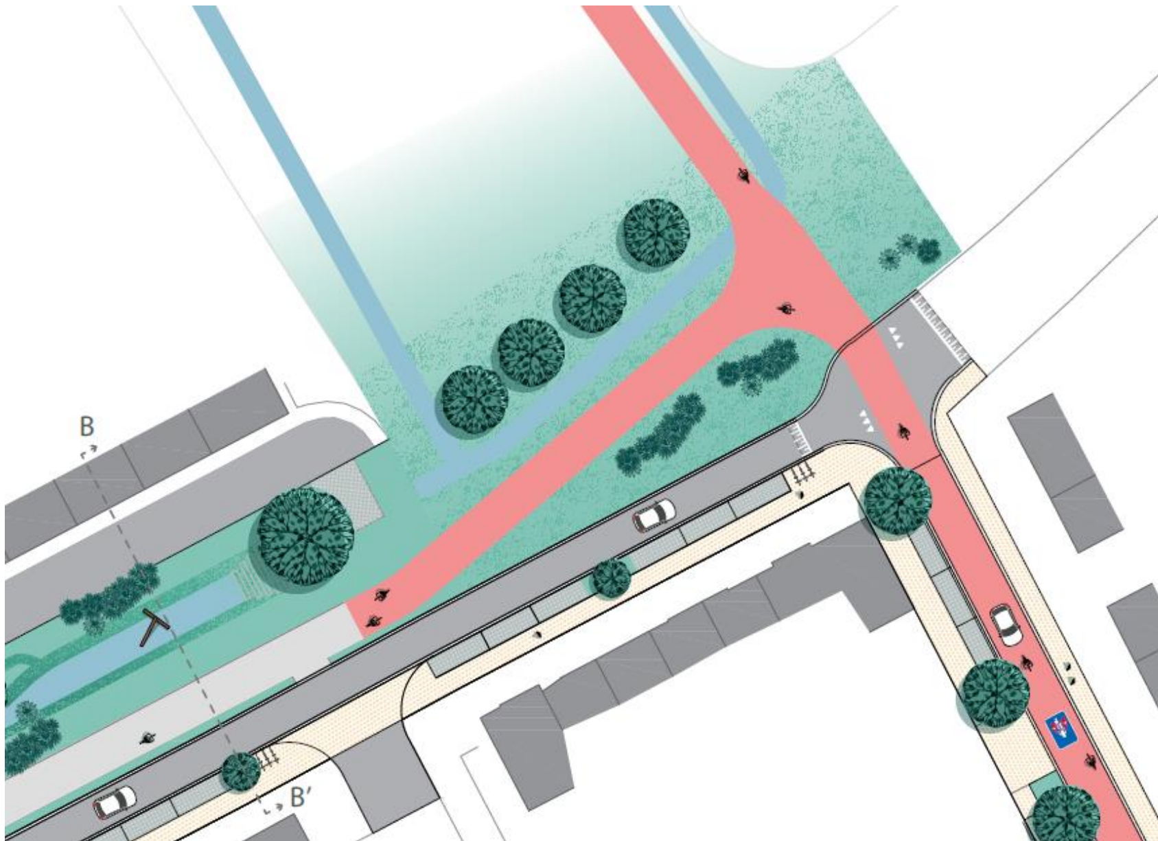
Aansluiting Molenstraat – Jakob Vandervaetstraat - N50c
